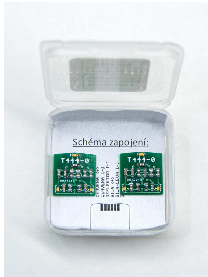
(a) Foto jednoho kusu čelního DPS
